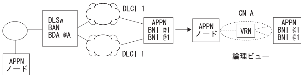
図7. BAN と複数のフレーム・リレー・ポートを使用する単一接続ネットワーク
