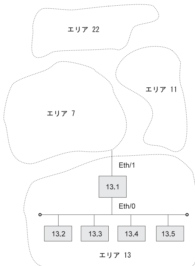
図 18. セキュリティ用のエリア・ルーティング・フィルターの例
