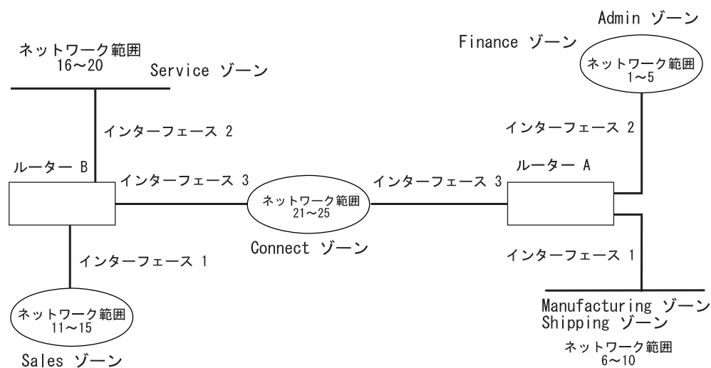
図13. ネットワーク・フィルターの例.
