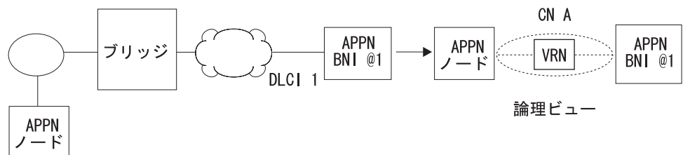
図 9.ブリッジングと 1 つのフレーム・リレー・ポートを使用する単一接続ネットワーク
